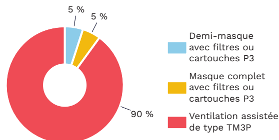
▲ Répartition des résultats par type de protections respiratoires
