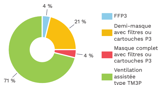
▲ Graphique 4 : répartition des résultats par type de protections respiratoires
